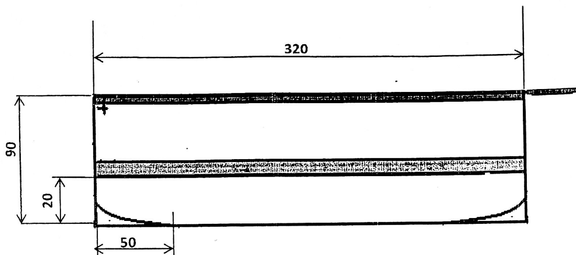
Рисунок 1 - технический рисунок подхвата для штор.
